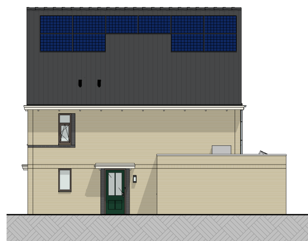
T44 rechtergevel (1:100)
