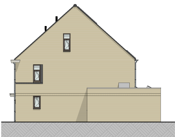
T40 rechtergevel (1:100)
