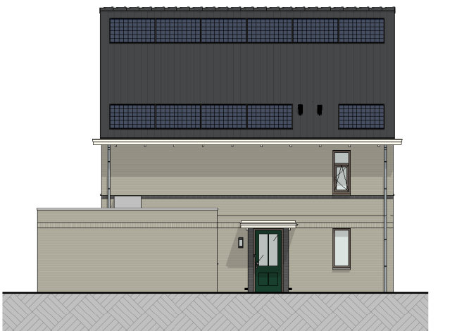
V32, V34, V35, V37 linkergevel (1:100)
