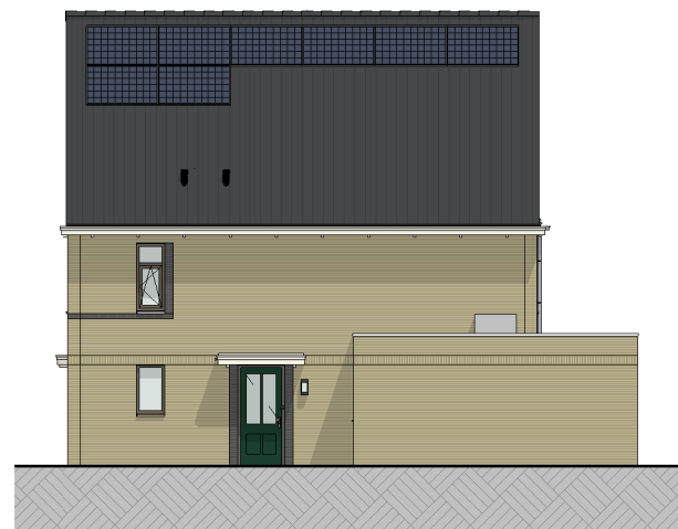
T31, T53 rechtergevel (1:100)
